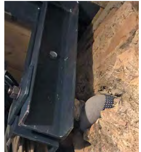
Vollständig verpresstes Ankerstrumpfsystem
